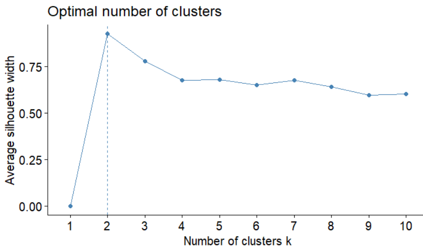
Gambar 9. rata-rata nilai silhouette coefficient dengan grafik
